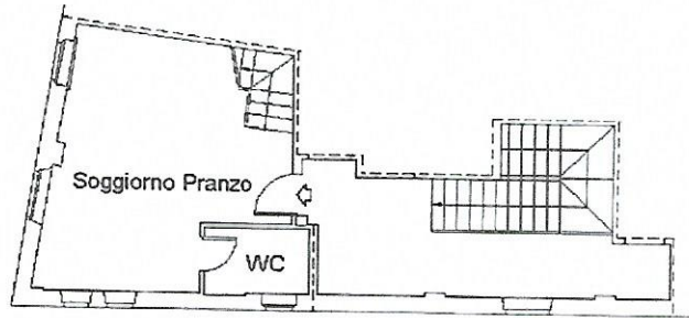
PIANO PRIMO h 2.80
