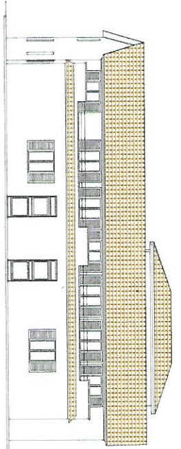
prospetto OVEST
